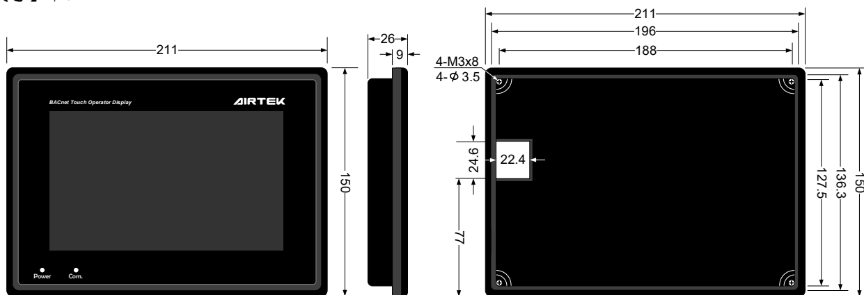
圖一、嵌燈式安裝示意圖
