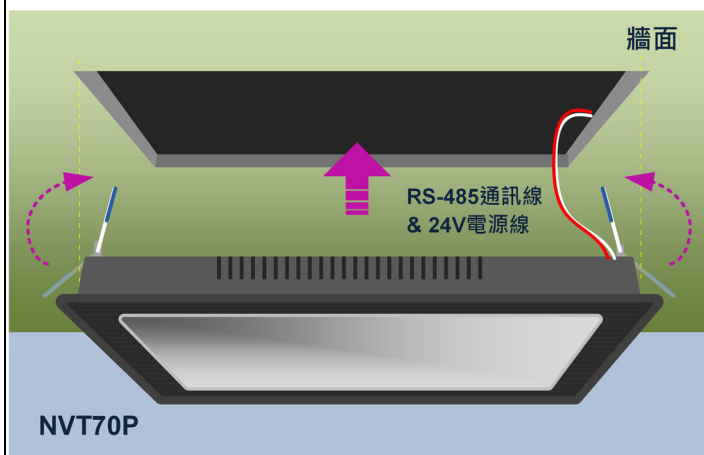
圖一、嵌燈式安裝示意圖
