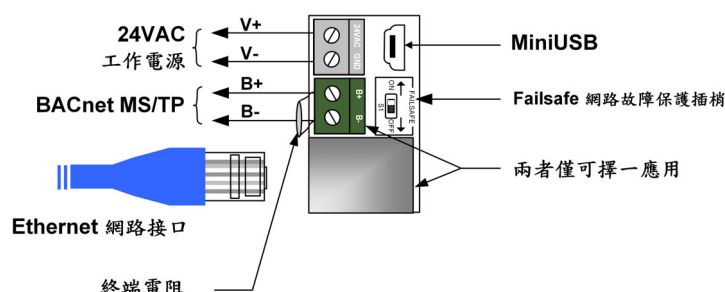
圖二、NVT70PE 接線
