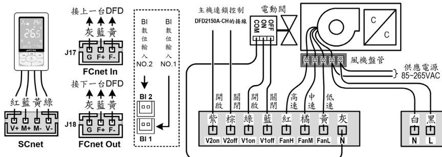
(圖三) DFD2150A-CH 控制接線圖
