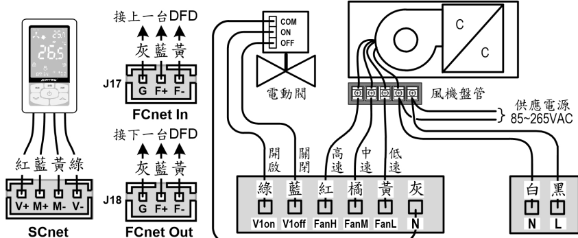
(圖一) DFD0140A 控制接線圖
