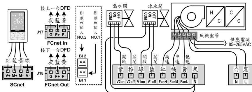
(圖二) DFD2150A 控制接線圖
