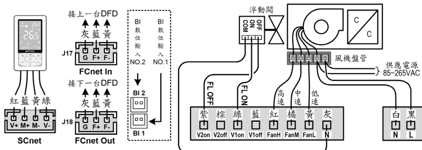
(圖四) DFD2150A-FL 控制接線圖
