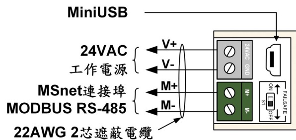
圖二、DST70P 接線
