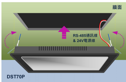
圖一、嵌燈式安裝示意圖
